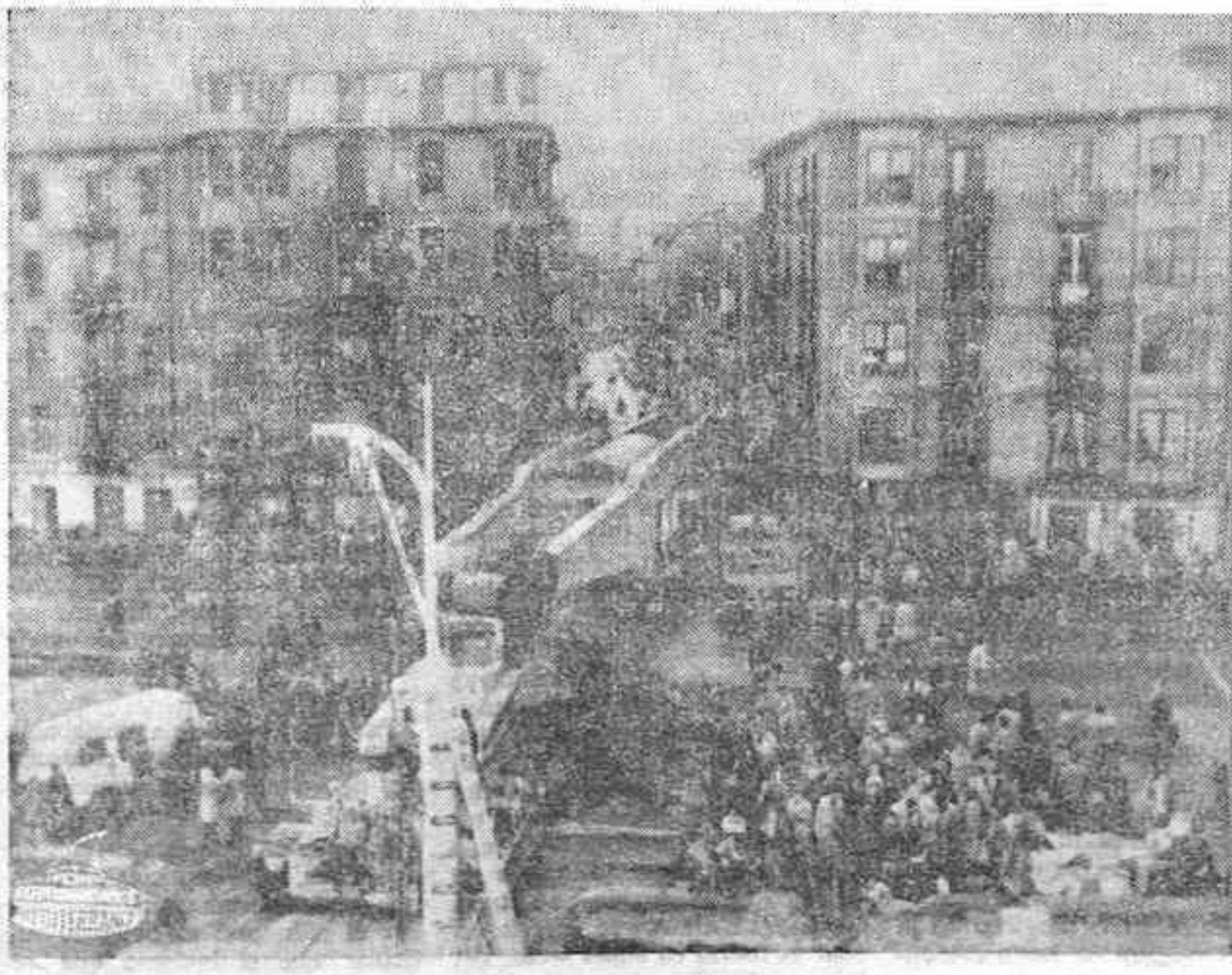
ERANDIO. — Estado en que quedó la cabina del convoy que transportaba el mayor turbogenerador para su embarque con destino a una central térmica española. A causa del vuelco, un operario resultó muerto y otros con heridas calificadas de muy graves. — (Telefoto Cifra Gráfica)
