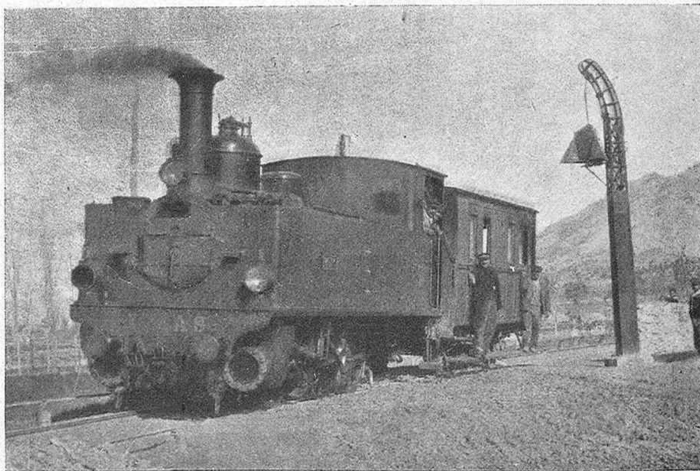
La locomotora en un paso á nivel.—Torre y campana sistema Basanta accionada automáticamente por las locomotoras minutos antes de pasar un tren.
