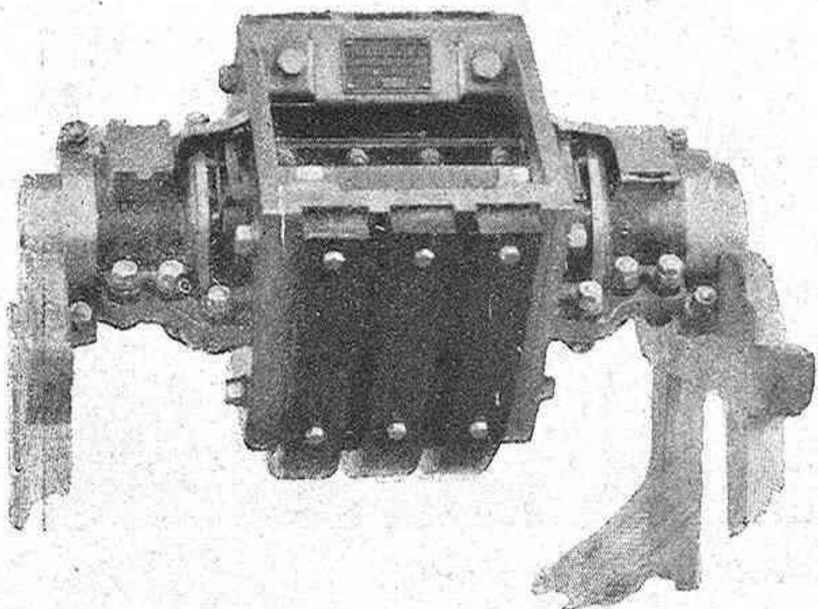
Máquina eléctrica, sistema Basanta, acoplada al eje de las locomotoras que tan excelente resultado han dado en las pruebas efectuadas últimamente en el ferrocarril económico de Villena á Yecla.
