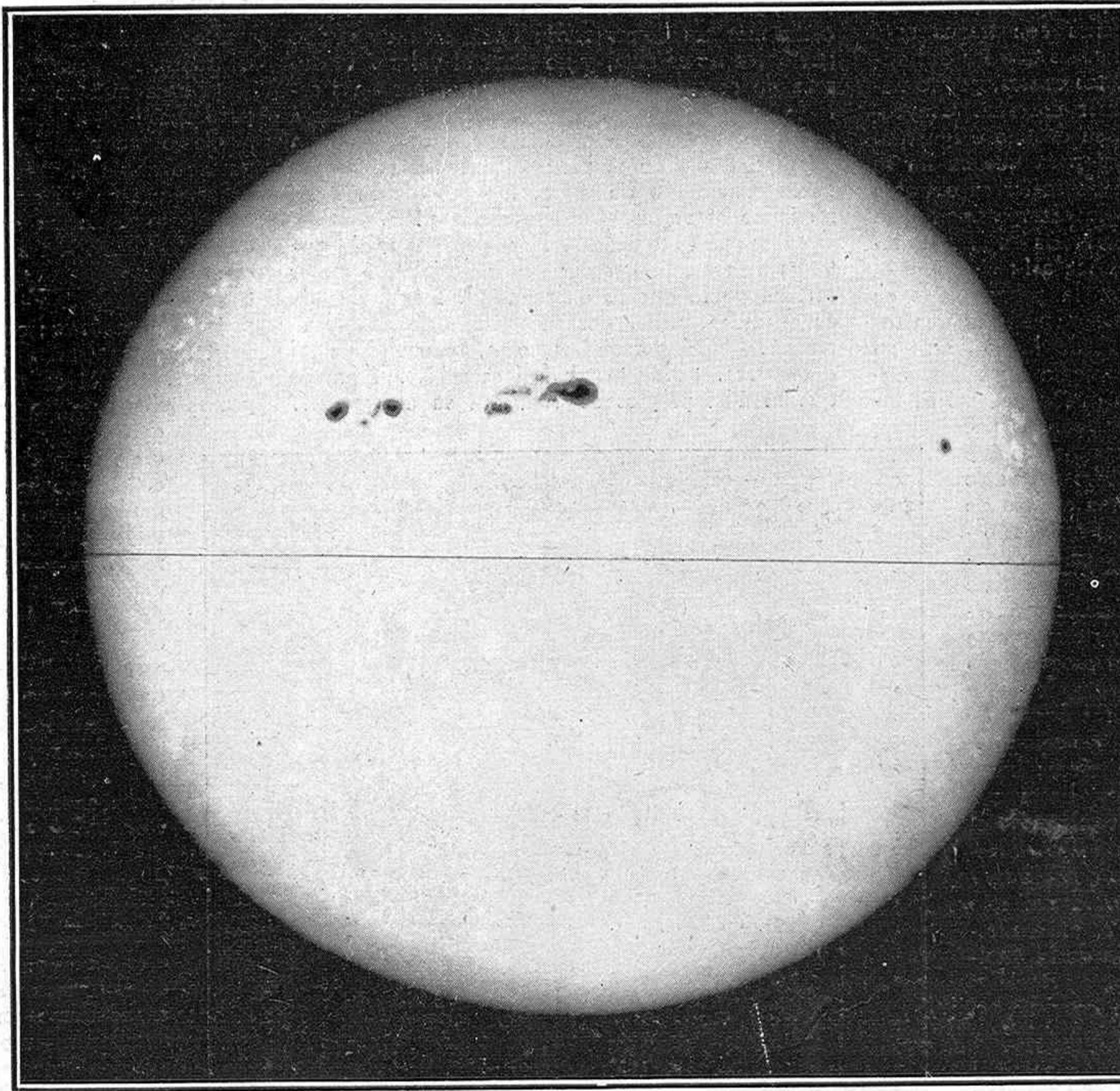
Fotografía del Sol obtenida en el Observatorio Astronómico de Madrid, con la ecuatorial de Stenheil, el día 3 de Enero de 1917, á las 10 h. 25 m. de la mañana, por el astrónomo D. Miguel Aguilar y Cuadrado
