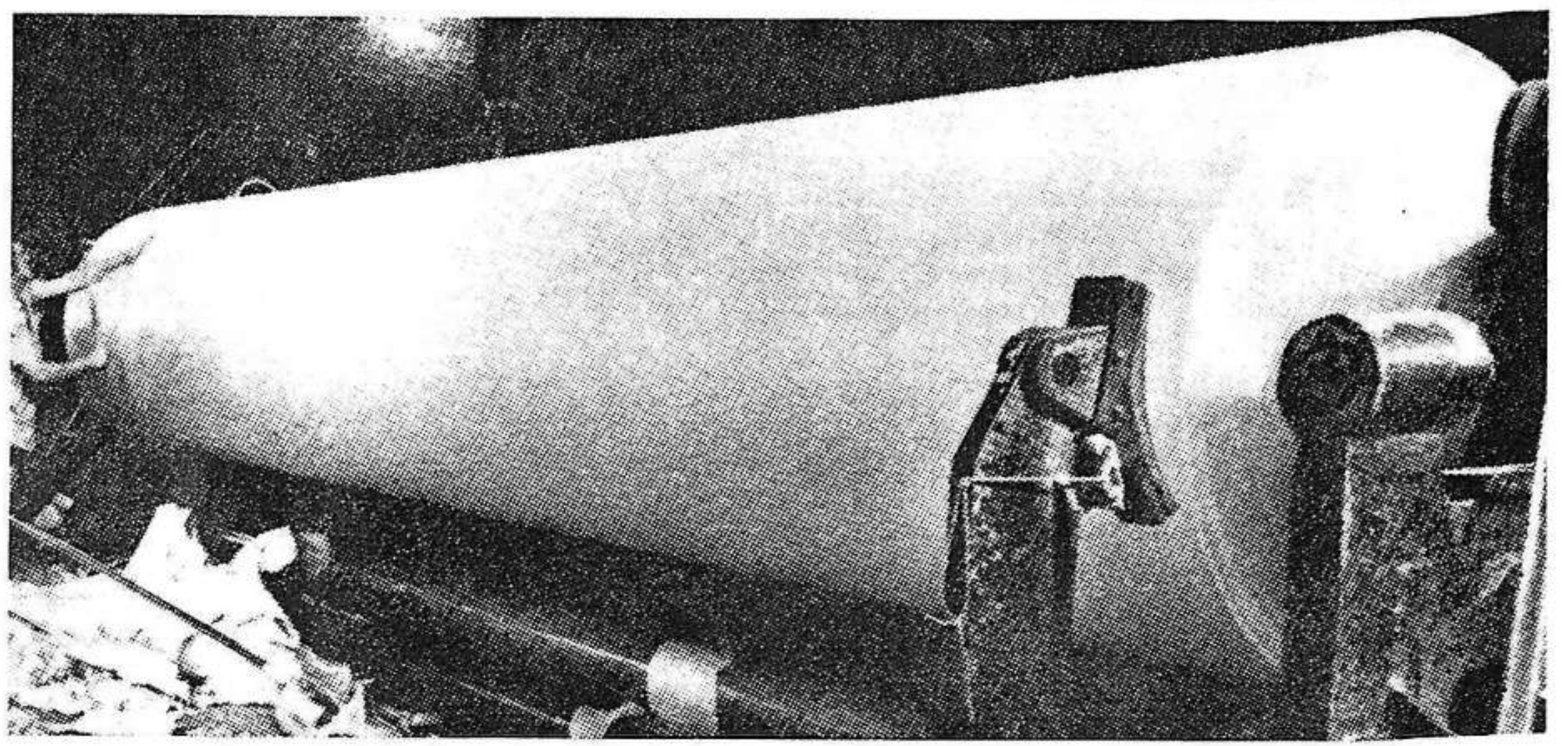
Un rollo de papel de 10 toneladas sale cada 40 minutos de la mayor máquina para papel periódico de Francia. La máquina tiene 97 m de largo; la cinta de papel circula a la velocidad de 42 km-hora.
