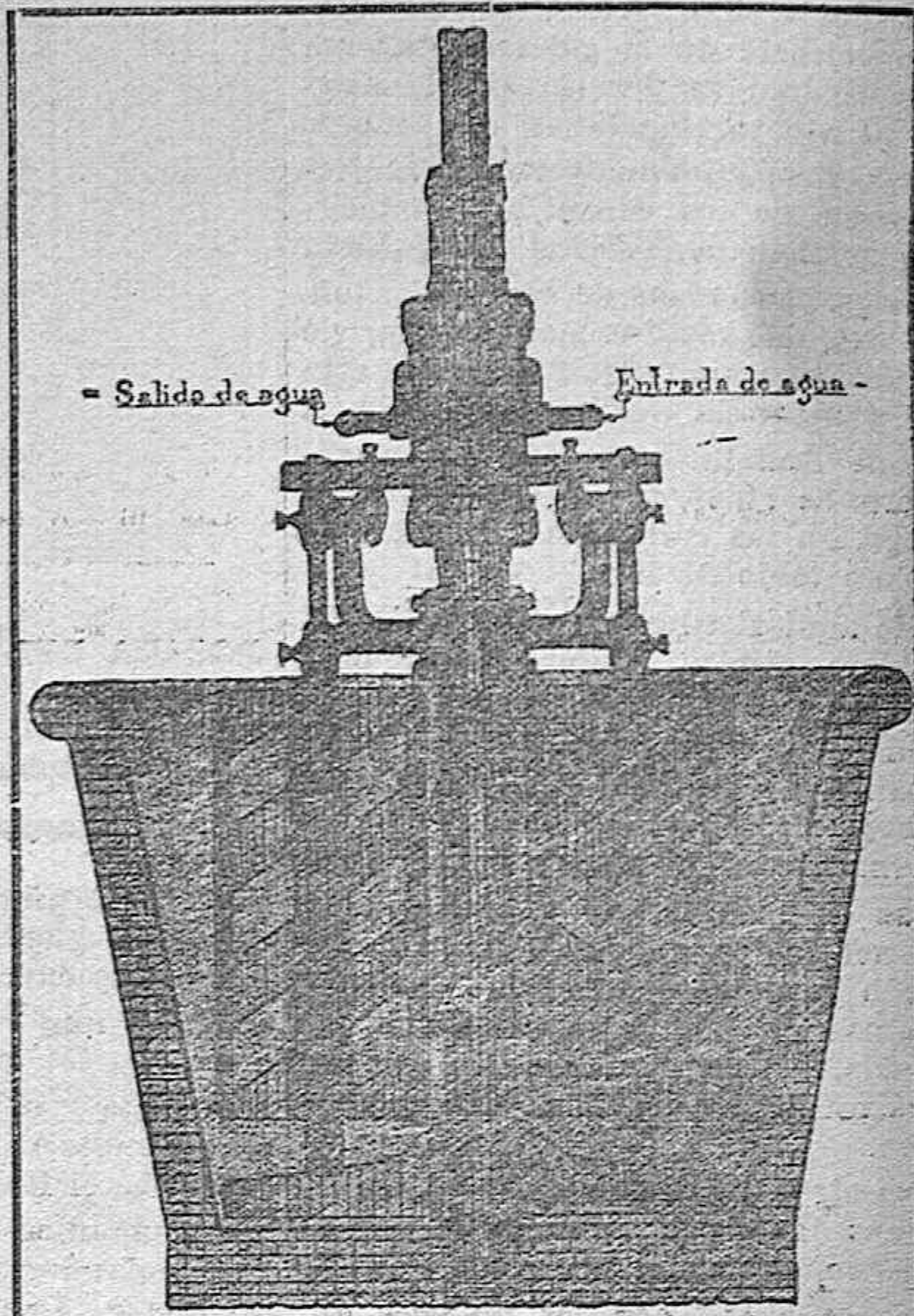
Una vista de mi batidora sin piedras y con dispositivo especial de calefacción en sus paletas y soporte central patente 131.064
