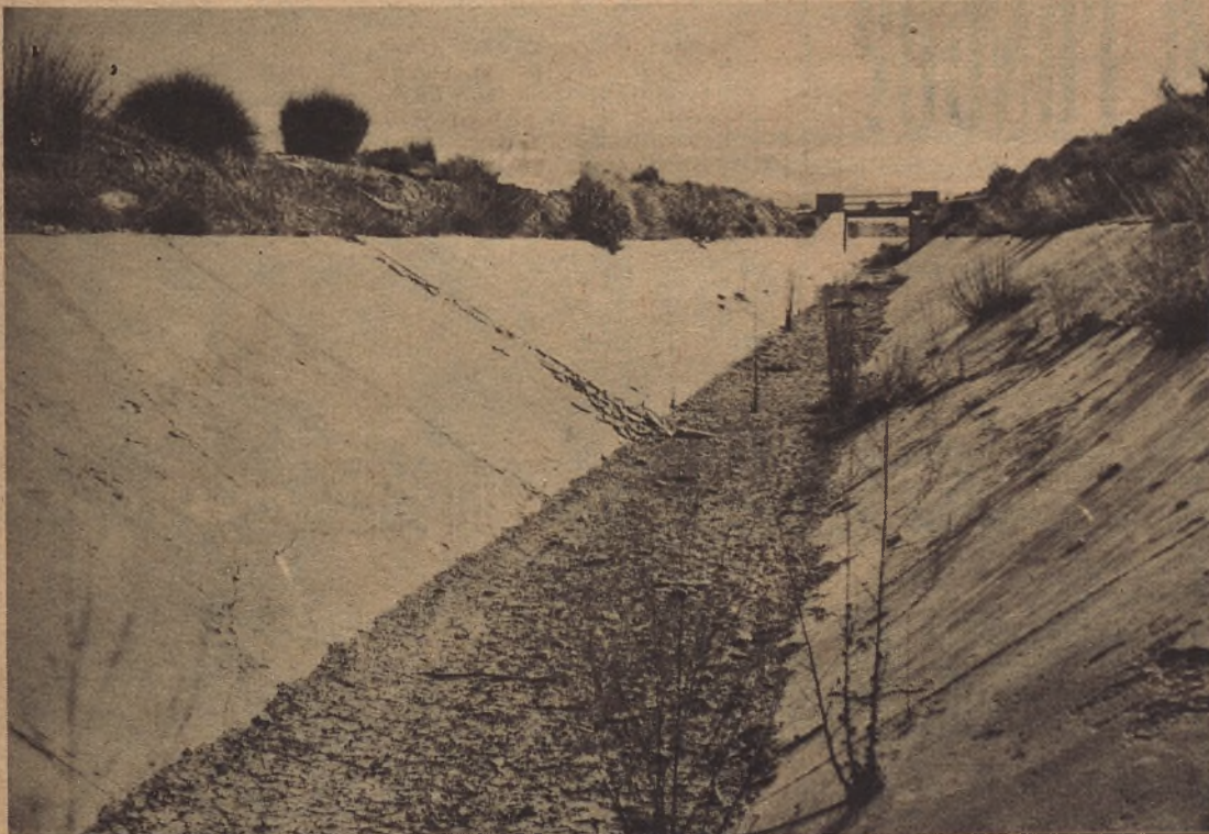
Estado actual de la acequia de la margen izquierda del Guadalope, construida en la época en que ocupaba la cartera de Obras Públicas el general Vigón, que poco a poco se va desmoronando sin que por su cauce haya discurrido una gota de agua.
