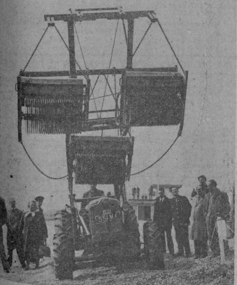
Este equipo fue expuesto recientemente en funcionamiento, en una demostración en Brighton, de métodos para eficiente limpieza de playas. En la práctica, las ruedas dentadas del equipo marchan sobre la playa, levantando a su paso cualesquiera depósitos de alúminas sólido que la marea haya depositado
