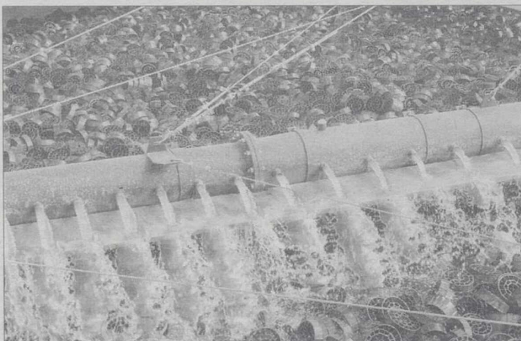
Tanque de filtros de una depuradora. / C.L.
