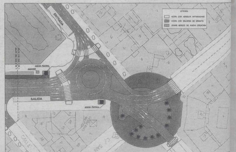
Plano del proyecto de rediseño de la plaza de Gabriel Lodares.
