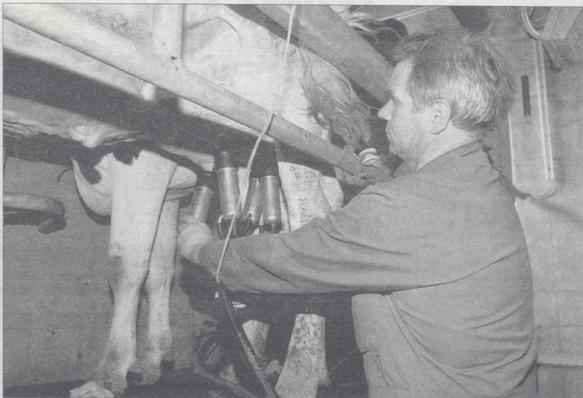
Ordeñado mecánico en una explotación ganadera. / FOTO: EC
