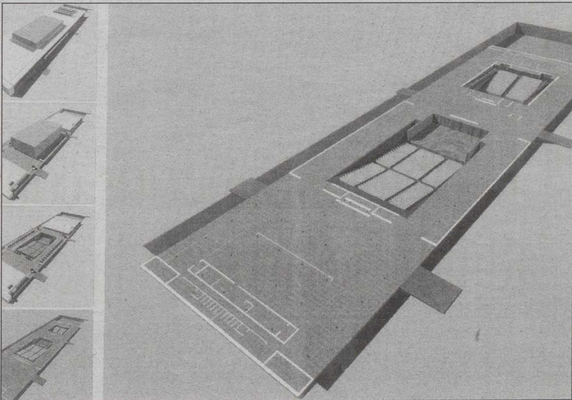
Plano del anteproyecto de Palacio de Congresos de Albacete.
