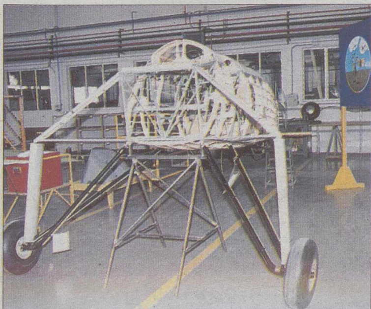
Aspecto del autogiro en fase de construcción.
