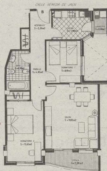
Vivienda tipo "B" Superficie útil=64,65m2 (planta 1)
