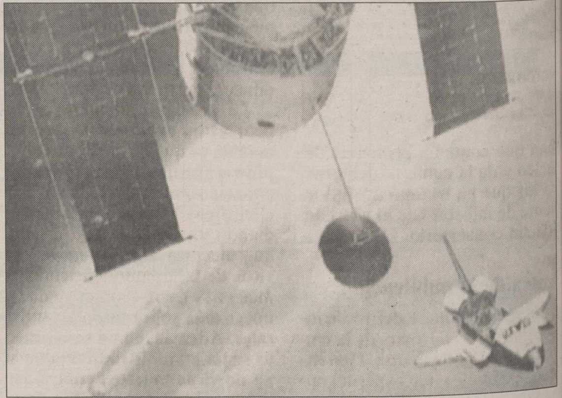
El supertelescopio espacial "Hubble" confirmó por primera vez la existencia de un monstruoso agujero.
