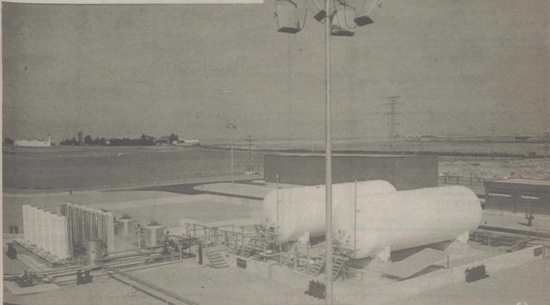
Planta de regasificación de gas natural (Polígono Industrial Campollano, AB)
