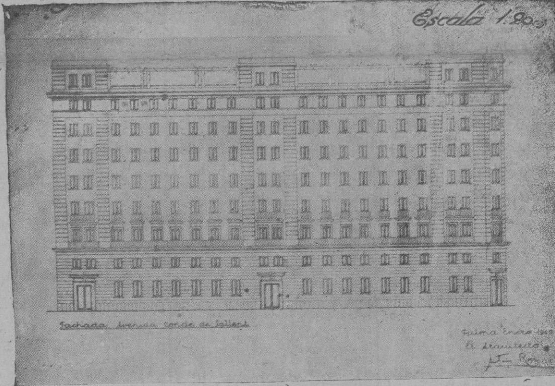
Grupo de viviendas protegidas que el Ayuntamiento de Palma acordó ayer construir para funcionarios, en la Avenida del Conde de Salent. Proyecto del Arquitecto don Antonio Roca
