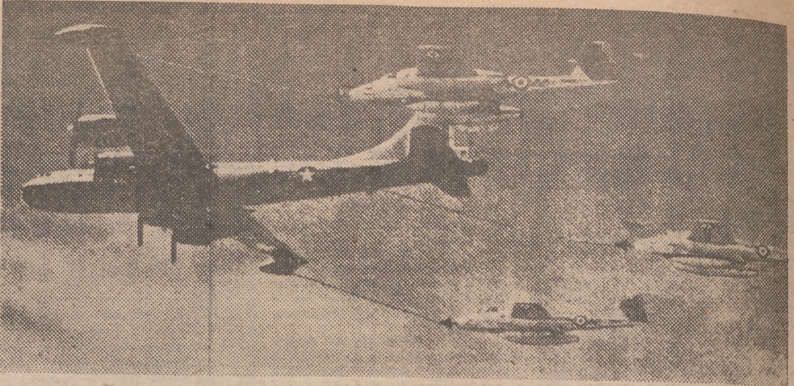
Un avión cisterna norteamericano "KB-29", abasteciendo de carburante, en pleno vuelo, a tres cazas a reacción ingleses "Meteors"
