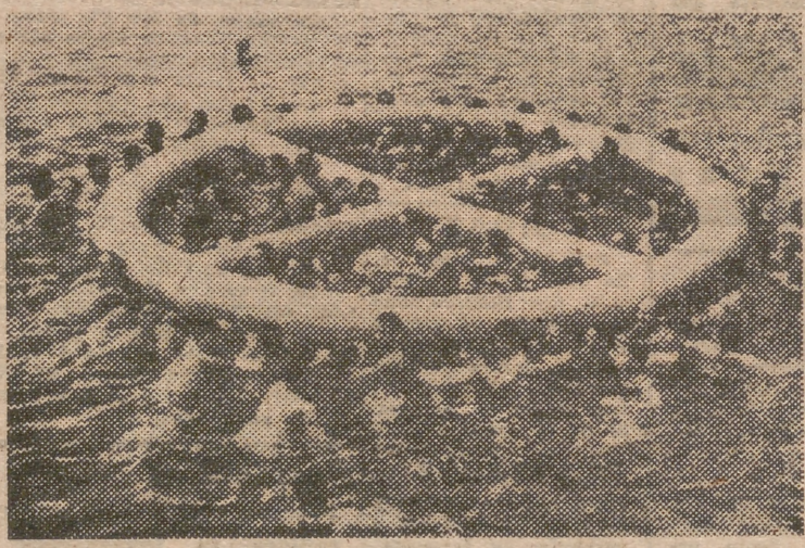
Un gigantesco salvavidas, de 38 pies de circunferencia y que pesa solamente 79 libras ha sido ensayado por la fuerza aérea de los Estados Unidos, con resultado ilustre. Cada salvavidas es capaz para cien hombres
