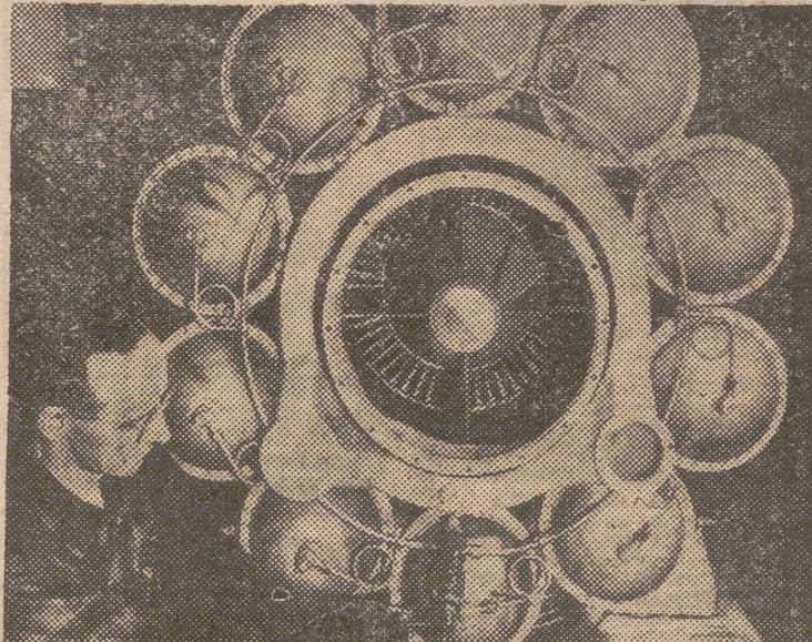
El nuevo motor de propulsión por reacción, producido por la «General Electric Company», en el que se aprecia la turbina que gira a más de 10.000 revoluciones por minuto a una temperatura superior a 815 grados centígrados
