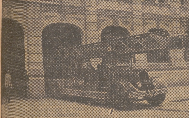
El gigantesco auto-escala, cuya escalera, desmontada, puede alcanzar la altura máxima de 50 metros
