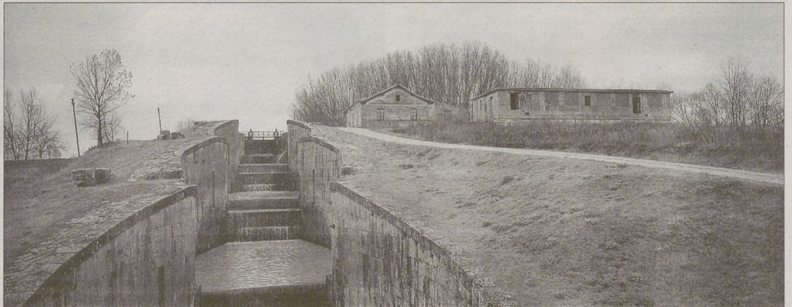
A la entrada de Frómista (Palencia) existe un impresionante grupo de cuatro esclusas que salvan un desnivel de 14 metros en el Canal de Castilla. / E. MARGARETO (ICAL)
