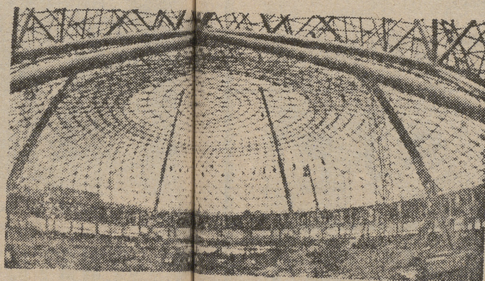
Una vez elevado el cuerpo de montadores proceden a la sujeción definitiva. En tanto, la estructura depende solamente de las grúas.
