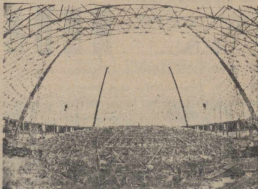
Concluido sobre el suelo el montaje de la zona central, se inicia la elevación mediante cuatro grúas telescópicas.
