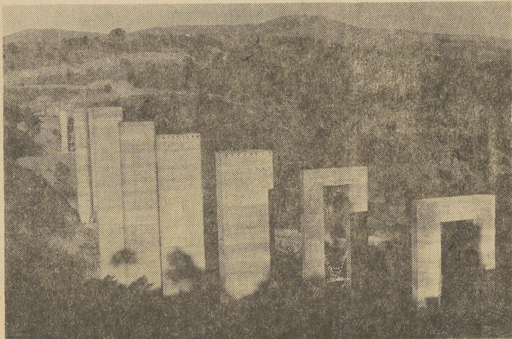
Una vista del viaducto que se construye sobre el río Cofio. Las enormes columnas, las más altas cuentan sesenta y tres metros y ocho de anchura. La obra va muy adelantada.
