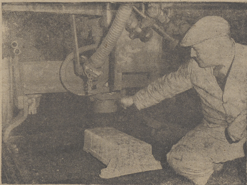
Primer trozo de control automático para la seguridad de trenes que se instalará en breve en la línea meridional de los Ferrocarriles Británicos. En esta fotografía, el montador jefe indica el receptor de una locomotora que acciona los imanes conectados eléctricamente con las señales de la vía. En el centro de la vía se ve claramente la caja de electroimanes.
