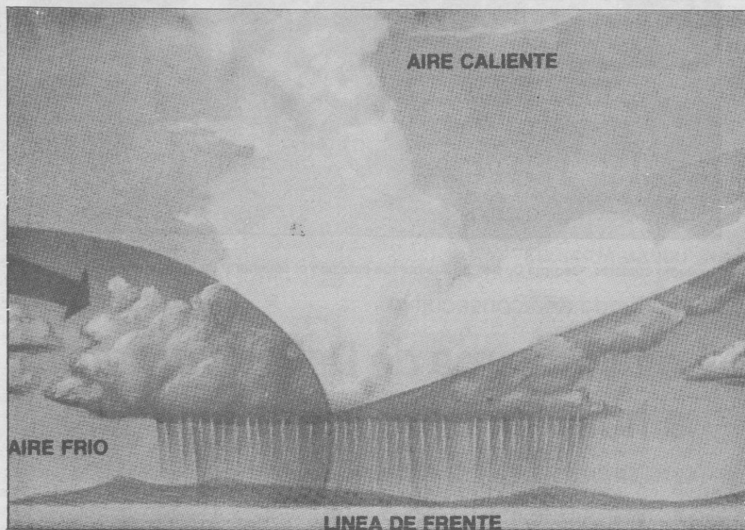
Encuentro de dos masas de aire en el ámbito de la oclusión.
