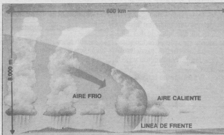
Esquema de frentes fríos y cálidos.
