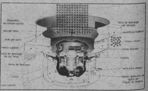
Esquema del separador Sweco
