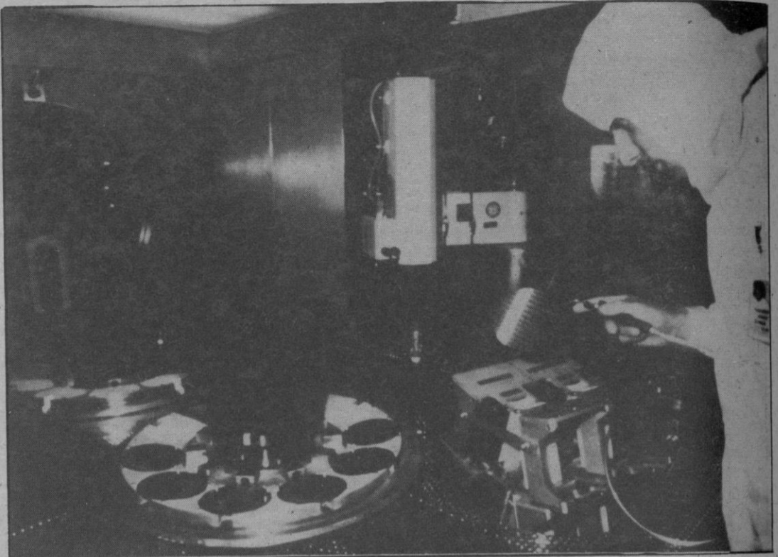
El primer «chip» de un megabitio producido recientemente en la planta que la multinacional IBM tiene en las cercanías de Stuttgart (Alemania Occidental). El tamaño de este nuevo «chip» el de mayor capacidad fabricado hasta el momento, es de 10,5 x 7,7 milímetros. En la foto, la producción de las piezas básicas, casi microscópicas, de silicio.—(Foto EFE)
