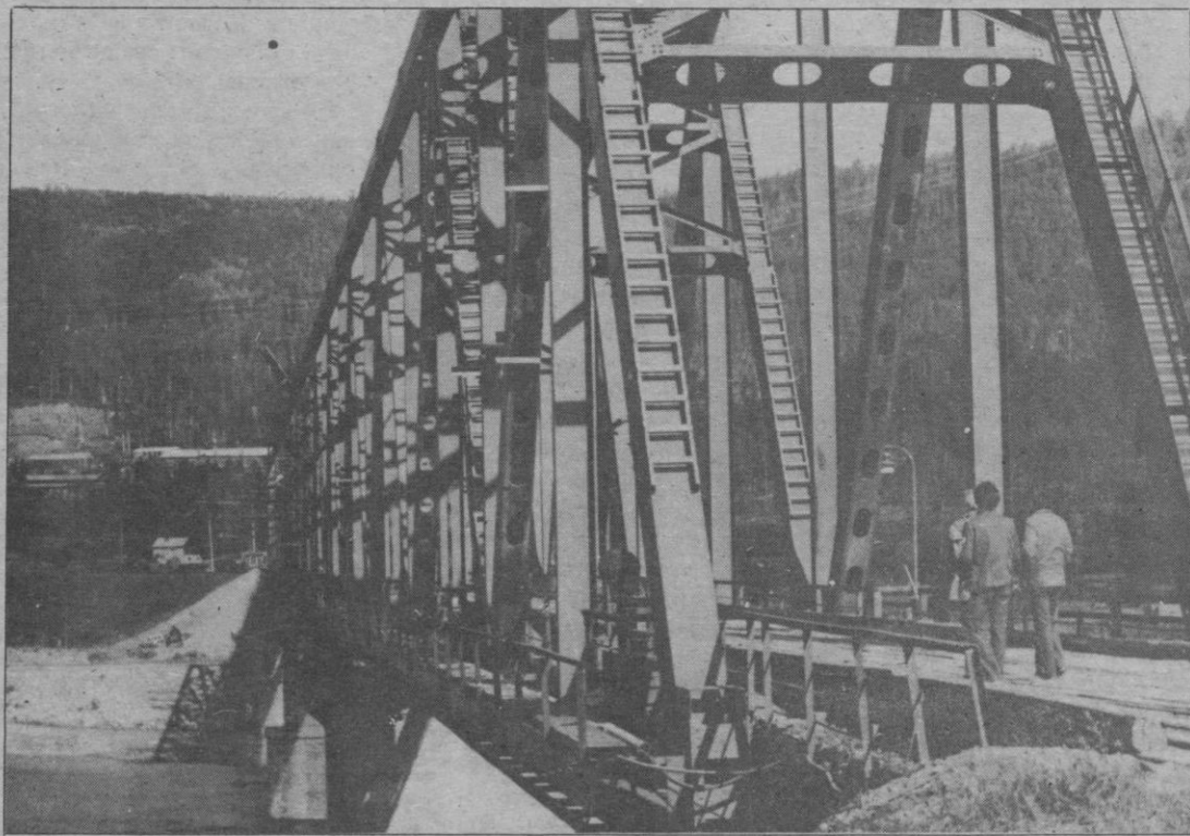
Puente a través del río Lena en la parte occidental del ferrocarril Baikal-Amur. —(Foto SP 83-472)
