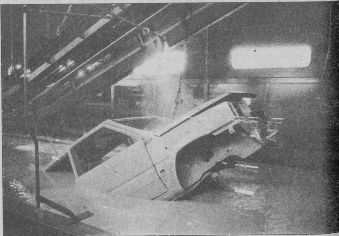
Uno de los procesos de fabricación del Panda: la pintura de cataforesis por inmersión
