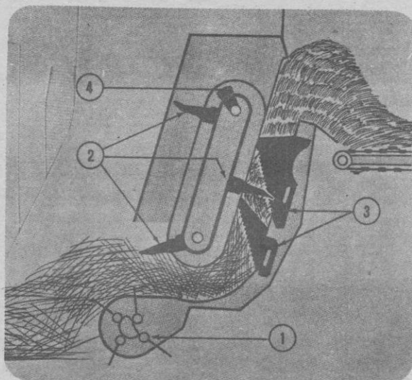
Esquema del sistema de recogida y elevación.
