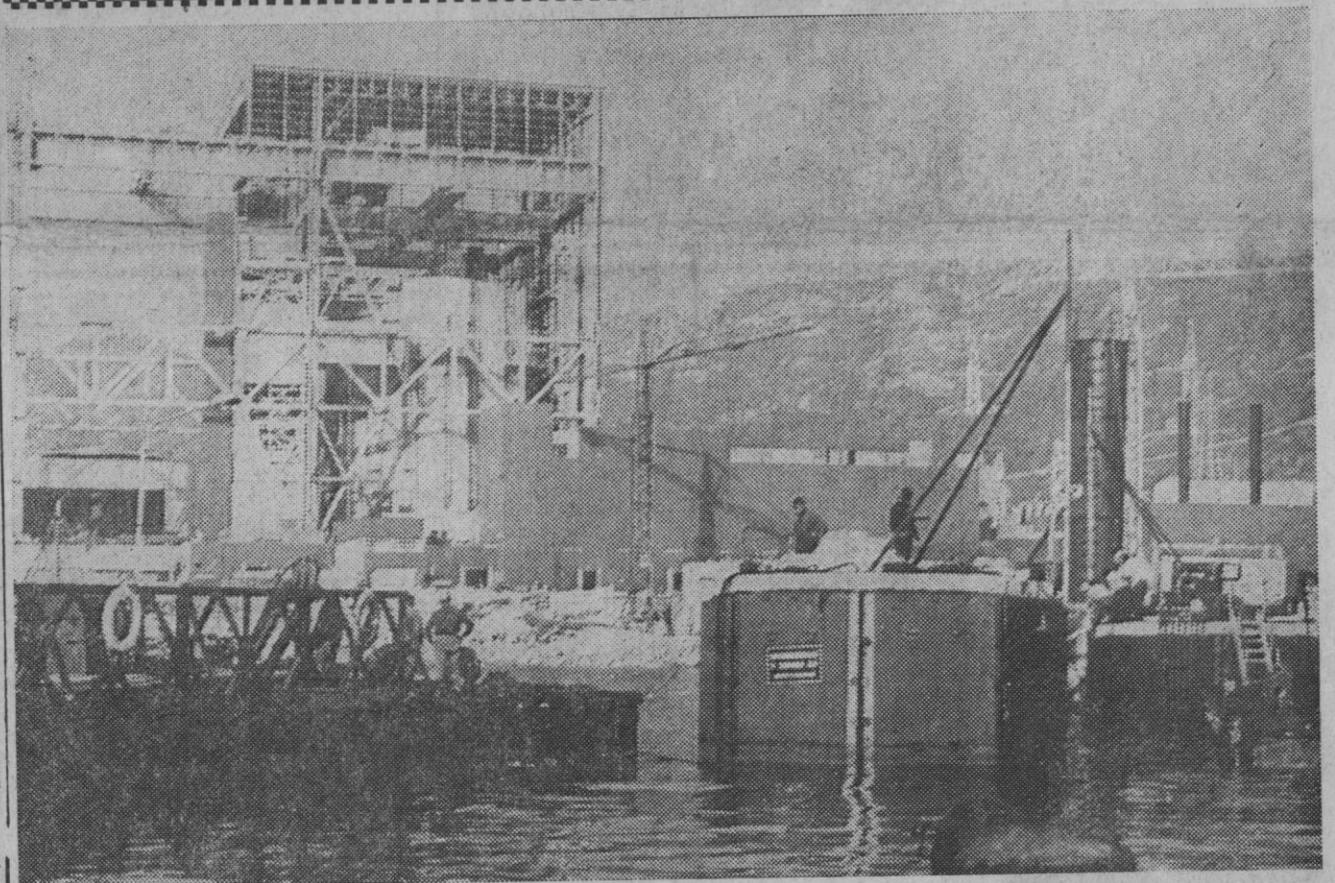
Tarragona.—Una vista de los trabajos de la central nuclear de Vandellós (Tarragona), que se encuentra en avanzado estado de construcción y será inaugurada en septiembre de 1972. Ahora se han iniciado los trabajos de carga del reactor nuclear.—(Foto Europa Press).
