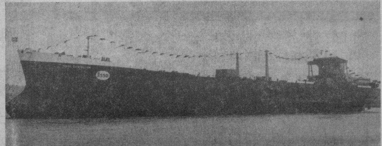
El Ferrol del Caudillo.—El petrolero «Esso-Castellón», considerado como el de mayor tonelaje de su clase en España, después de su botadura en los astilleros ferrolanos. El nuevo petrolero desplaza noventa y tres mil toneladas, mide doscientos cuarenta y cuatro metros de eslora por 38,10 de manga y 16,60 de puntal, y su tripulación es de sólo veintisiete hombres.—(Foto Europa Press.)
