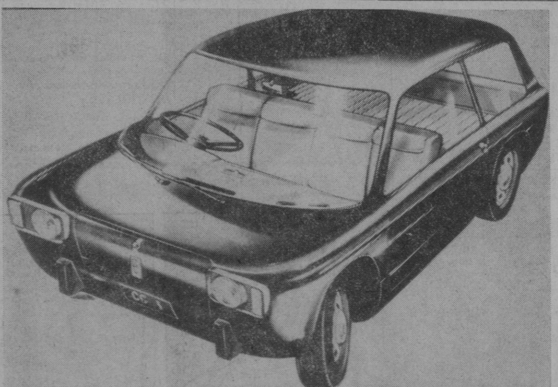
Londres.—El Carter Coaster, coche eléctrico inventado por el ingeniero de cincuenta años Alistair Carter. El coche es un cuatro asientos, con carrocería de plástico, motor eléctrico trasero, alimentado por cuatro baterías de doce voltios de las que se utilizan generalmente en los coches de motor de gasolina.—(Foto Europa Press.)
