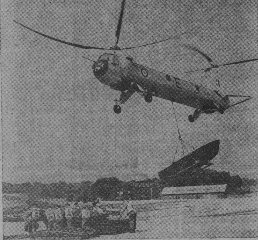
Ingenieros del Ejército británico se disponen a construir un puente flotante, con motivo de una reciente demostración de técnicas y equipo de ingeniería militar. Contrariamente que el tipo viejo de puente de pontones, que había de ser transportado por camiones, las nuevas técnicas permiten usar pontones livianos, que pueden portarse con helicópteros
