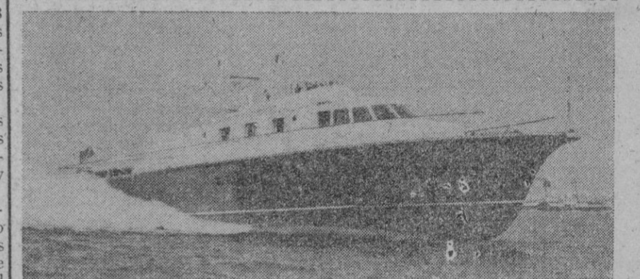
El "Mercury", yate construido en Portsmouth, para el naviero griego señor Stavros Niarchos, es tenido por el más veloz yate privado que hay en el mundo, pues tres turbinas de gas Bristol Siddeley "Marine Proteus" le permiten alcanzar velocidades de más de cincuenta nudos, sin ningún equipo auxiliar de propulsión. El "Marine Proteus", versión marítima del aeromotor que propulsa los aviones "Britannia", tiene una turbina autónoma de fuerza, y es tan regulable, que se puede emplear en las maniobras lentas. Entre las muchas ventajas de estos motores figuran su poco peso y volumen, su falta de vibración y la gran velocidad que proporcionan.
