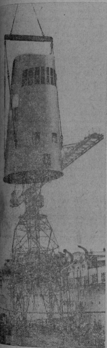
Construcción de una chimenea especialmente diseñada a la cubierta superior del nuevo trasatlántico británico «Empress of Canada», que ha costado ocho millones de libras, en un taller inglés. La chimenea, que pesa sesenta y cuatro toneladas, fue levantada por una gigantesca grúa en un espacio de 15 metros sobre el terreno. La chimenea, de 13,71 por 7,13 metros en la base y 15,24 de altura, ha sido especialmente diseñada para librar de humo al barco.
