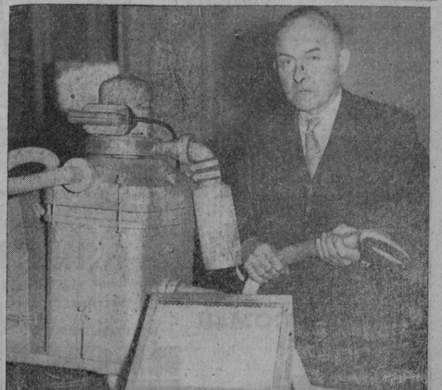
Aspiradora-pulimentadora que filtra los microbios recogidos del suelo y los destruye. El invento eliminará una de las causas principales de las re-infecciones que ocurren en los hospitales. A diferencia de la aspiradora doméstica normal, ésta aspira los microbios a través de dos mallas superfinas, garantizando que éstas captarán partículas de bacteria de una diezmilésima de milímetro. La máquina sirve también para aspirar el polvo radiactivo
