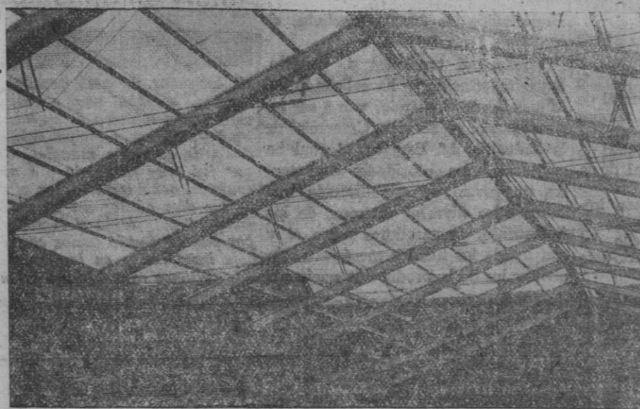
Detalle parcial de la cubierta «Z» de 13,40 metros de luces y 35 de longitud, realizada en esta capital bajo la dirección del arquitecto municipal don Francisco Fernández Vega.
