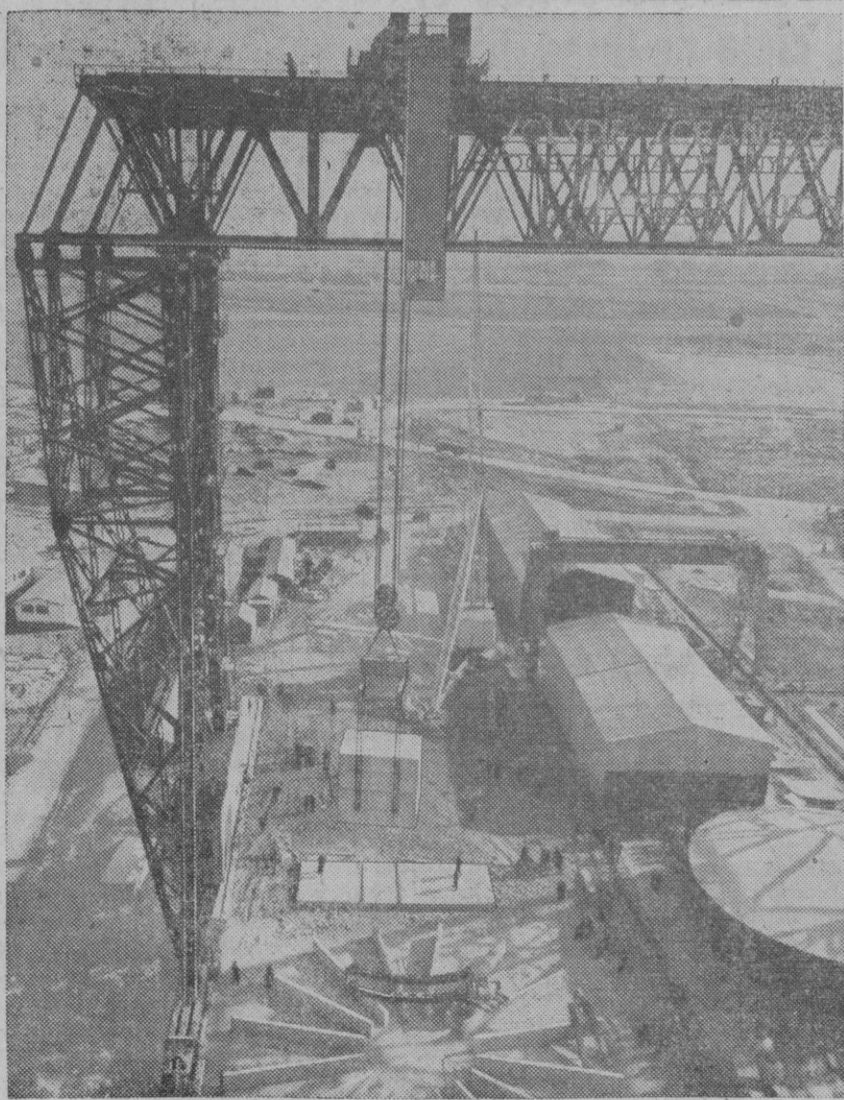
En la construcción de la central electroatómica de Bradwell (Essex), se ahorra tiempo y dinero con el empleo de esta enorme grúa de 55,5 m. de altura, que es el mayor de su tipo en el mundo. Esta grúa, llamada Goliat, abarca los edificios del reactor y está montada sobre ocho trenes articulados de cuatro ruedas, pudiendo transportar calderas pesadas o estructuras del reactor de 200 toneladas de peso a una gran altura sobre el solar de construcción y colocarla en posición en los reactores sin interrumpir los trabajos en otros edificios. La grúa Goliat, contiene 700 toneladas de acero y 13.000 tuercas y pasadores
