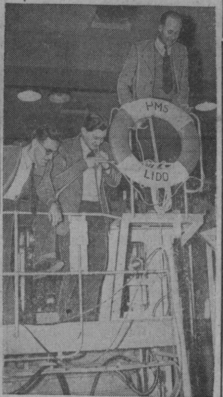
Recientemente se demostró en el Establecimiento de Investigaciones sobre la energía atómica, de Harwell, un nuevo reactor del tipo de «biscina». El cinturón salvavidas que cuelga del costado no tiene otro objeto que el de agregar un detalle marítimo. En esta fotografía, tomada desde cierta altura, aparecen en el alma del reactor varios técnicos que miran hacia abajo, a un gran tanque de agua purificada, en el cual se hallan en suspensión elementos de combustible de uranio enriquecido
