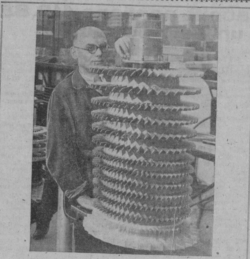
En la fotografía se ve a un técnico de una firma británica fabricante de motores de aviación montando un motor de turboreacción. Este motor es el "Proteus" del mismo tipo que el que impulsa al avión de pasajeros cuatrimotor Bristol "Britannia"
