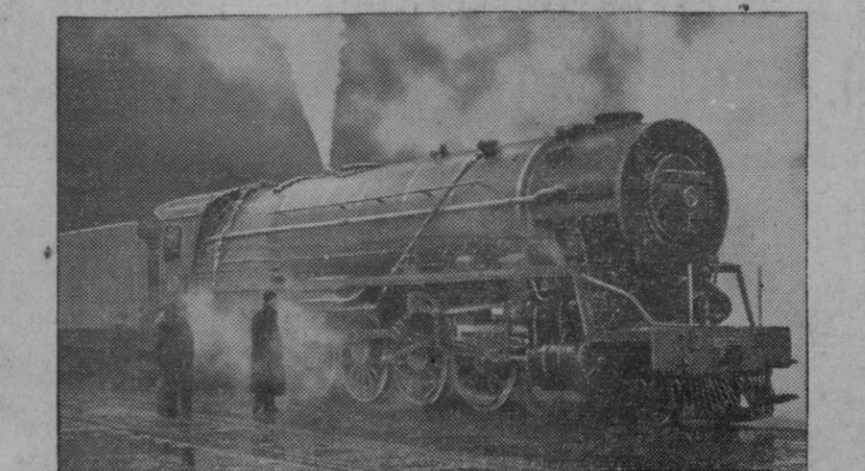
Una de las locomotoras que Gran Bretaña suministra a los ferrocarriles sudafricanos y que seguramente exportará también a Rusia. En orden de marcha, incluido el tender, pesa 181 toneladas
