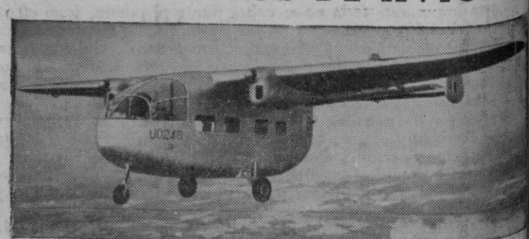
Fotografía de un aparato Miles Aerovan, que, como puede verse, es un aparato que goza de mucha visibilidad y comodidad. Tiene una velocidad de crucero de 110 millas por hora.
