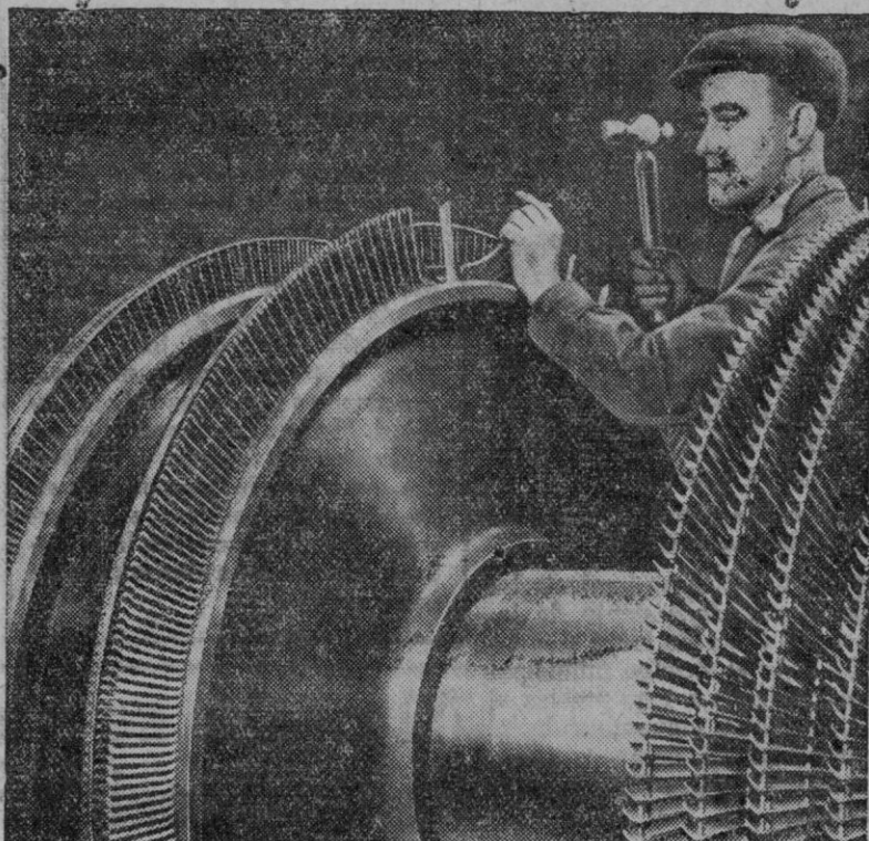
Instalación de las cuchillas de acero en la rota giratoria de un motor de turbina de vapor. La corriente de alta presión que pasa entre las cuchillas hace girar la turbina a más velocidad
