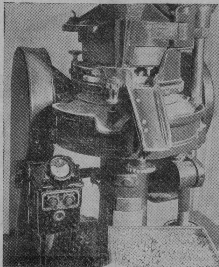
También en Inglaterra se fabrica intensivamente la "Mepacrina"—sustitutivo de la quinina, que ha hecho desaparecer casi los casos de paludismo—. La máquina representada en la fotografía produce 339 tabletas por minuto. La fábrica de "Mepacrina" suministra cuarenta millones de tabletas por semana
