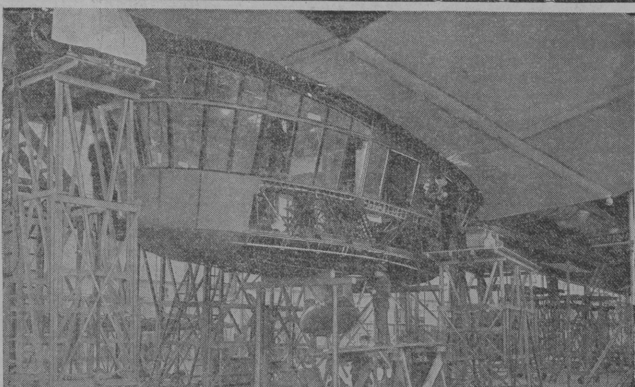
El dirigible alemán "L. Z. 129", cuya construcción pronto se terminará en los talleres de Friedrichshafen. Dicho dirigible, que será el más grande del mundo, emprenderá la ruta aérea de Europa a América del Sur, pudiendo transportar cincuenta viajeros y veinticinco toneladas de carga
