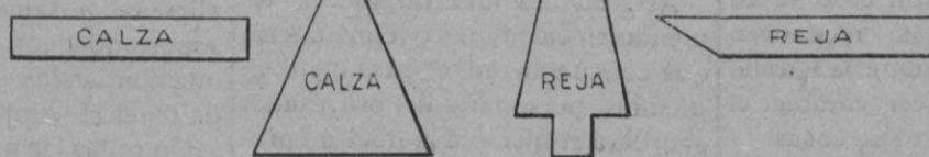
RECORTES Y PLETINAS PARA FABRICACION DE HERRADURAS
