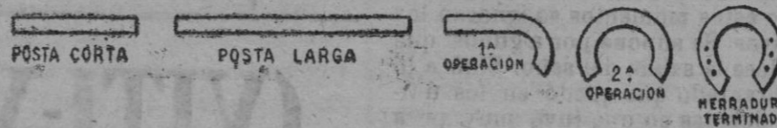
RECORTES Y PLETINAS PARA FABRICACIÓN DE HERRADURAS.
