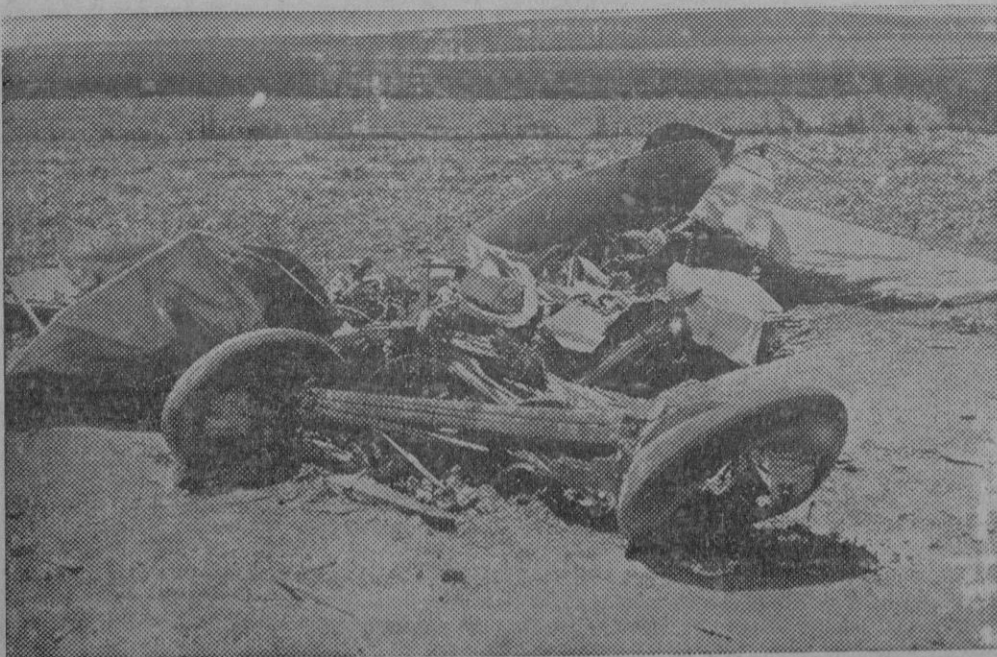
ACCIDENTE DE AVIACION (MADRID).—Estado en que quedó el avión al que se rompió un alerón cuando volaba a una altura de 2.300 metros el cual era tripulado por el teniente Joaquín Escribano y el teniente alumno Félix Alvarez. Sus tripulantes se arrojaron con paracaídas salvándose de una muerte segura.
