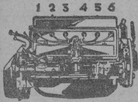
El motor de seis cilindros Chevrolet trabaja normalmente a 1.600 revoluciones por minuto
